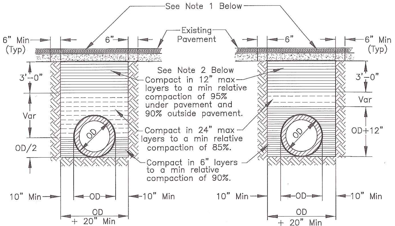
RIGID CONDUIT
